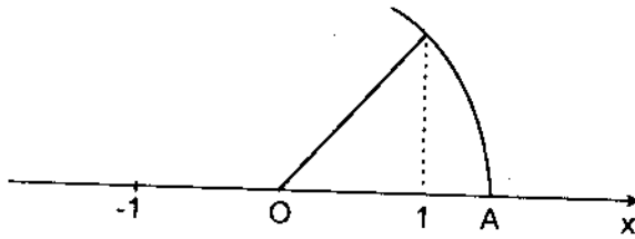
Hình 1.2. Điểm A ứng với số \sqrt{2}
